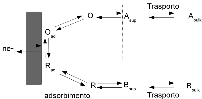
Figura 5: Generico processo elettrochimico
