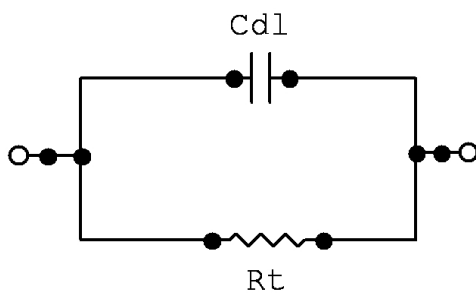
Figura 8: Impedenza dovuta al solo trasferimento elettronico
