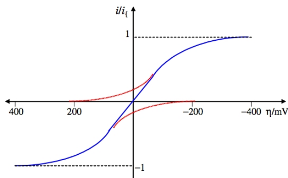
Figura 7: Corrente in funzione del sovrapotenziale
